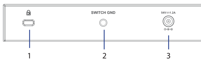
Figur 3: Kontakter på baksiden
