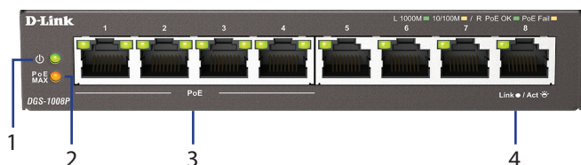
Rysunek 1: Kontrolki LED na panelu przednim
