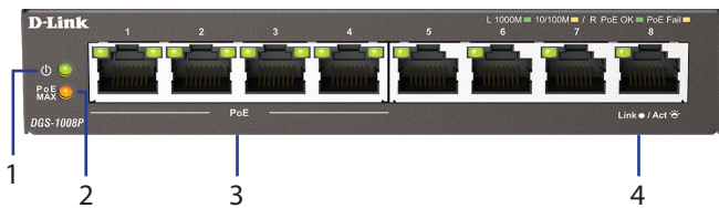
Abbildung 1: LEDs an der Vorderseite
