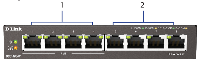
Kuva 2: Etupaneelin liittimet
