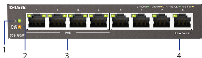
1. ábra: Az elülső panel LED-jei
