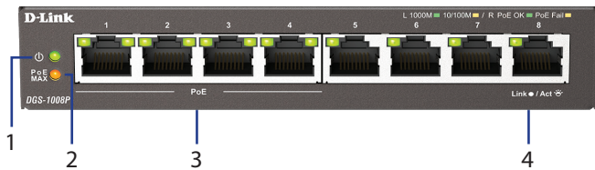
Kuva 1: etupaneelin LED-valot
