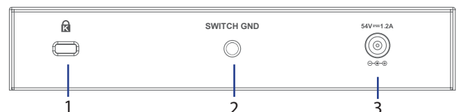
Kuva 3: Takapaneelin liittimet
