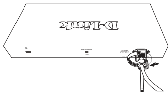
電源コードの周りに電源コード固定器具を巻きつける
