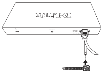
將固定器插入束帶
