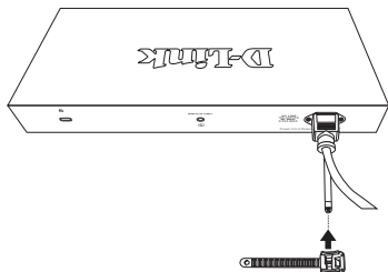
Conecte el retenedor a la abrazadera
