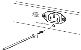
插入束帶
