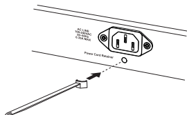
Установка стяжки
