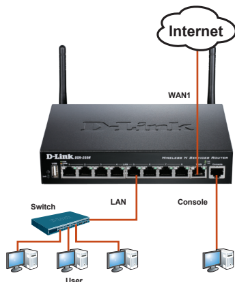
Figura 3: Exemplo de cabeamento básico
