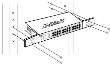
図3 スイッチをラックに取り付ける
