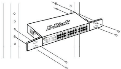
Gambar 3. Memasang switch ke rak dengan ukuran standar
