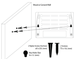
Abbildung 4. Desktop-Switch - Wandmontage
