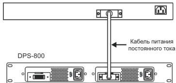
Задняя панель
