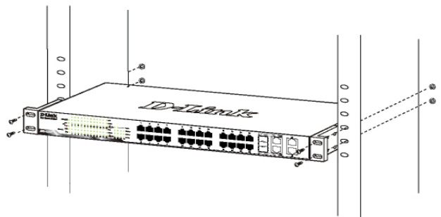
Gambar 3. Memasang switch ke rak dengan ukuran standar
