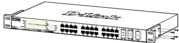
Abbildung 2: Einbauwinkel anbringen
