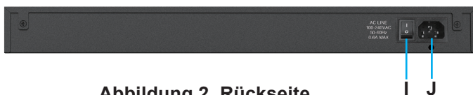
Abbildung 2. Rückseite
