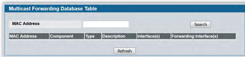
Figure 143: MFDB Table
